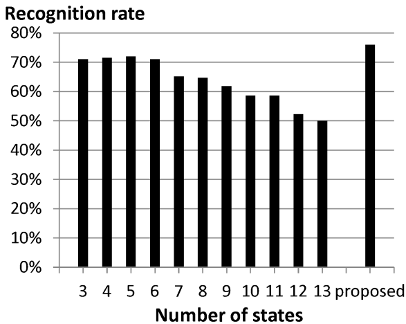
図 15 状態数固定と提案手法の認識率の比較
