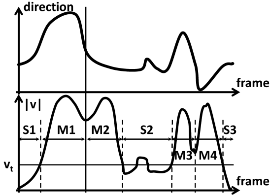
図 11 向きによる状態分割 Fig. 11 Division by the direction.
