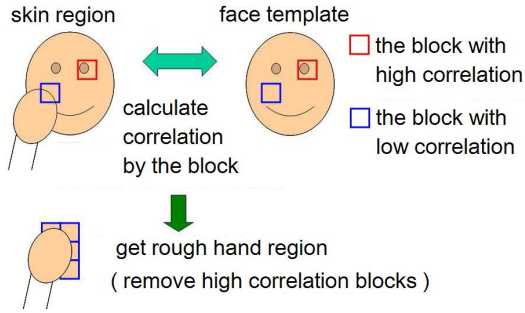
図4 相関を利用した顔領域の除去 Fig.4 Face removal by luminance correlation.
