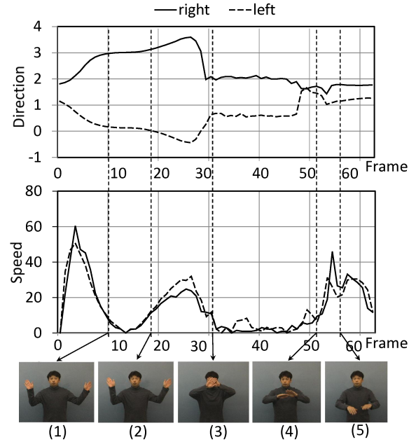
図 12 状態分割の例 Fig. 12 Example of state division.
