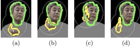
図 3 バックトラック有の場合の手領域抽出
